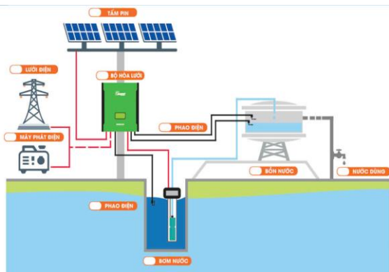
DÙNG KẾT HỢP ĐIỆN LƯỚI VÀ ĐIỆN MÁY PHÁT ĐIỆN
