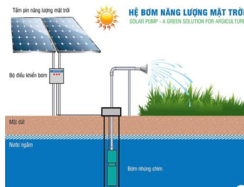
DÙNG ĐỘC LẬP CHO NHỮNG NƠI CHƯA CÓ ĐIỆN
